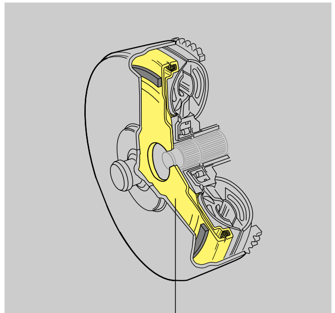
Wandlerüberbrückungskupplung
